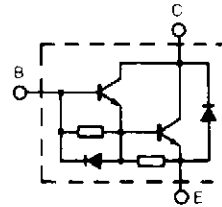
SOT-93
